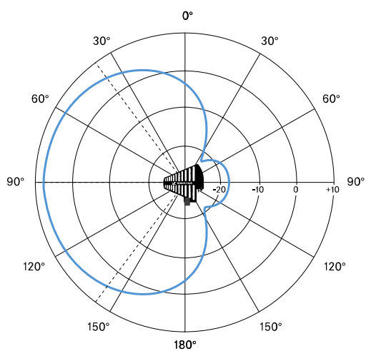
典型值极性特征图
