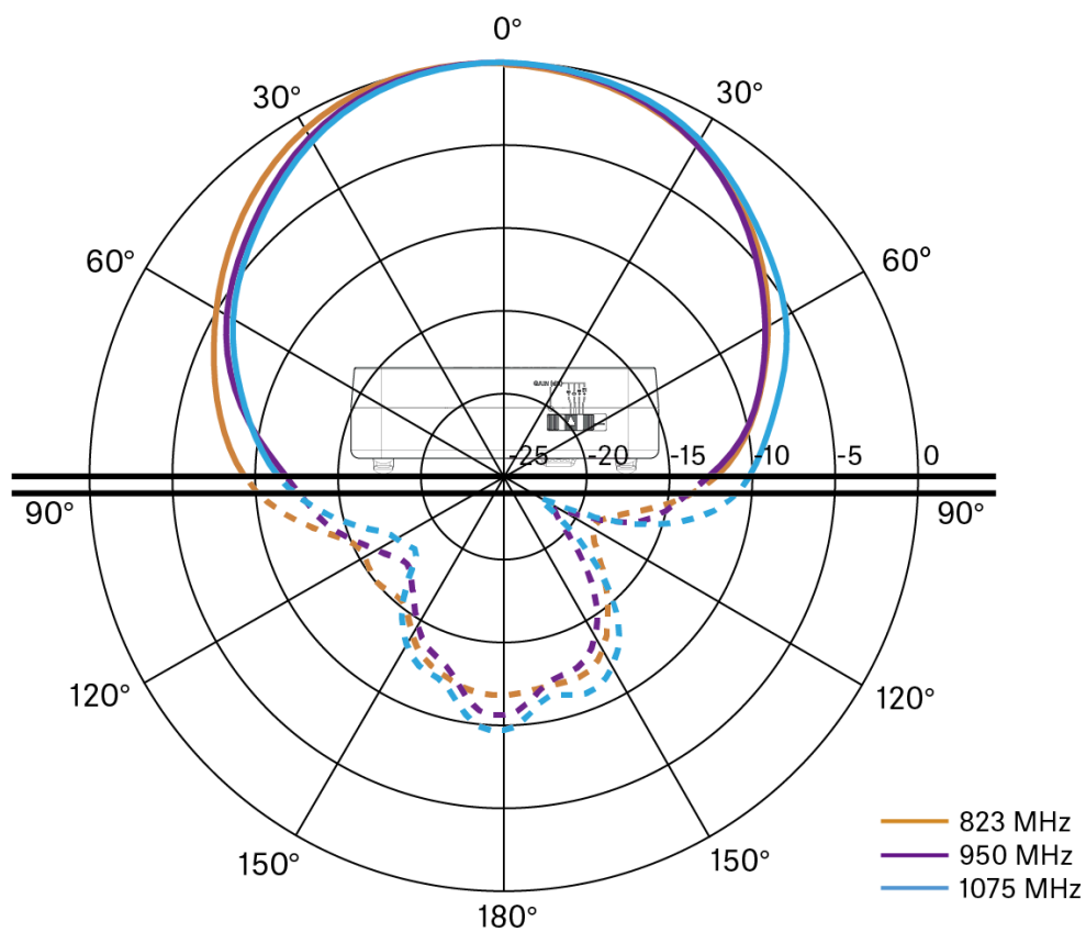
UHF (823-1075 MHz) 水平 [dB]
