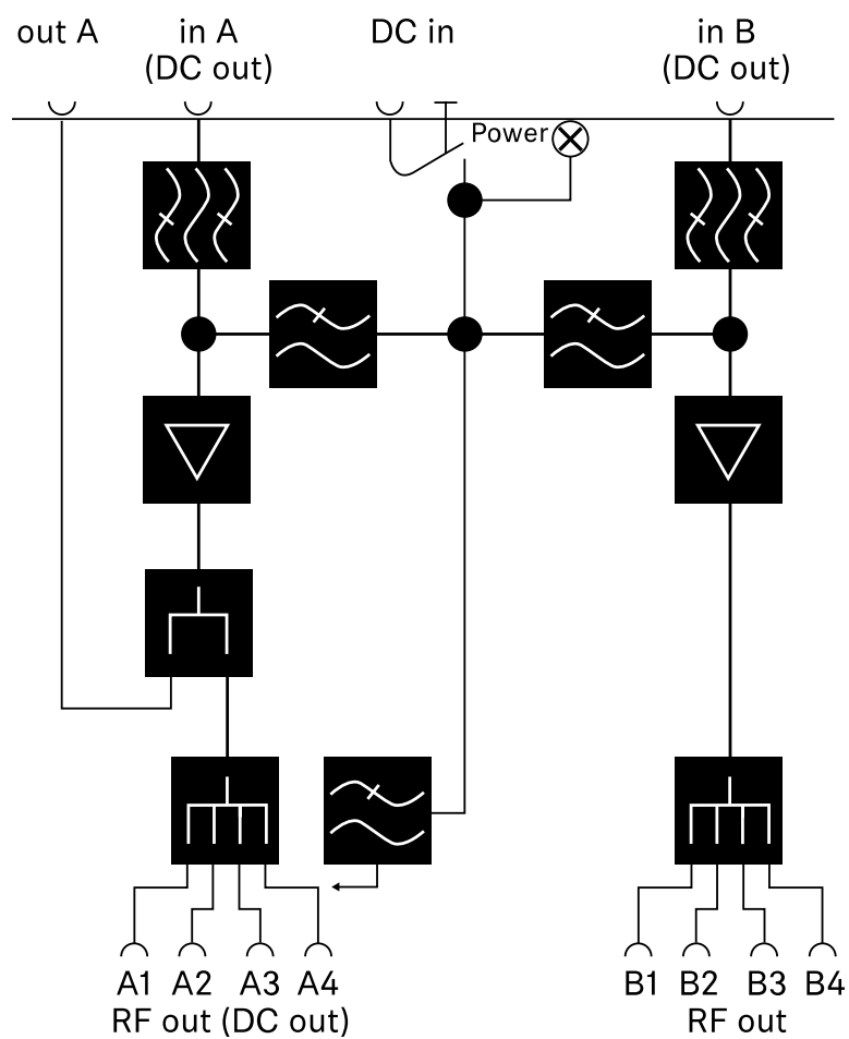
连接框图
