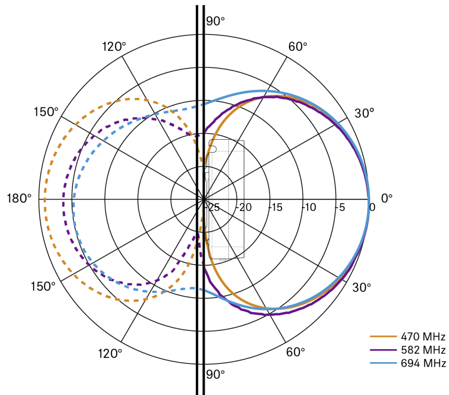
UHF(470-694MHz) 수평 [dB]
