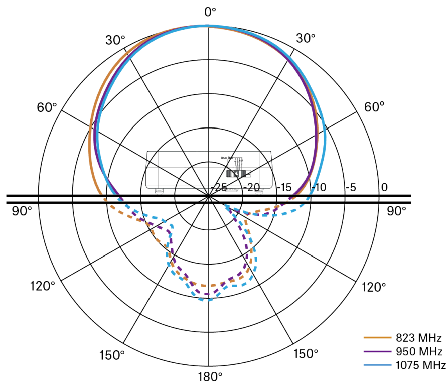
1G8 수직 [dB]
