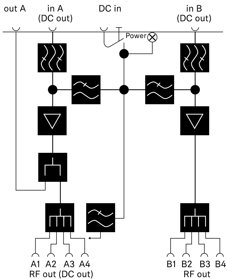
Diagrama de bloque
