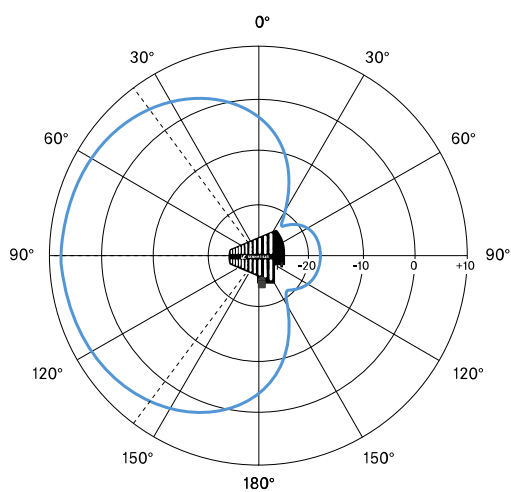
Diagrama de polaridad Diagrama polar
