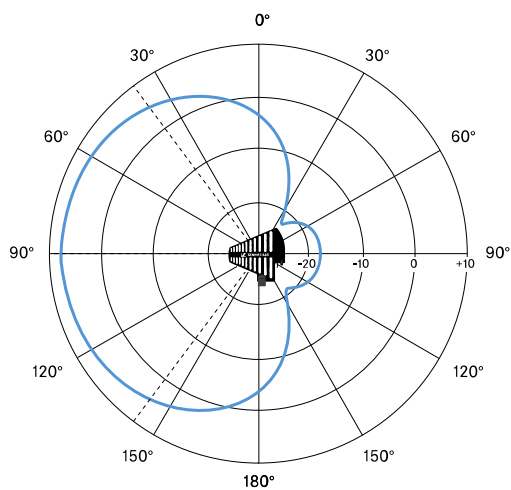
Typ. Polardiagramm
