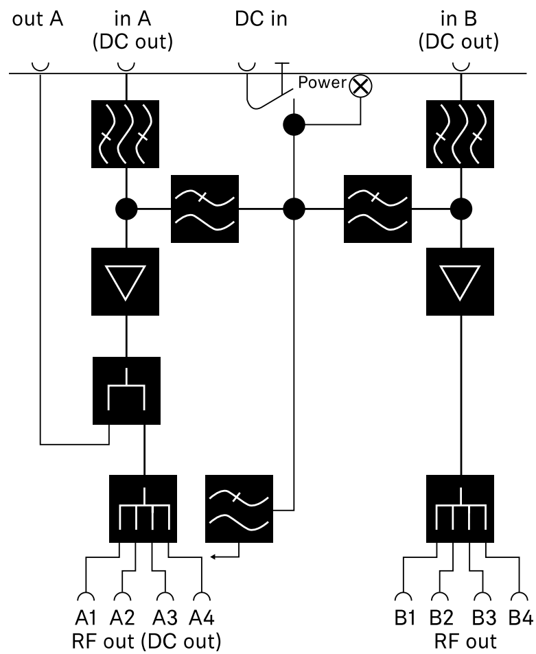
Blockschaltbild
