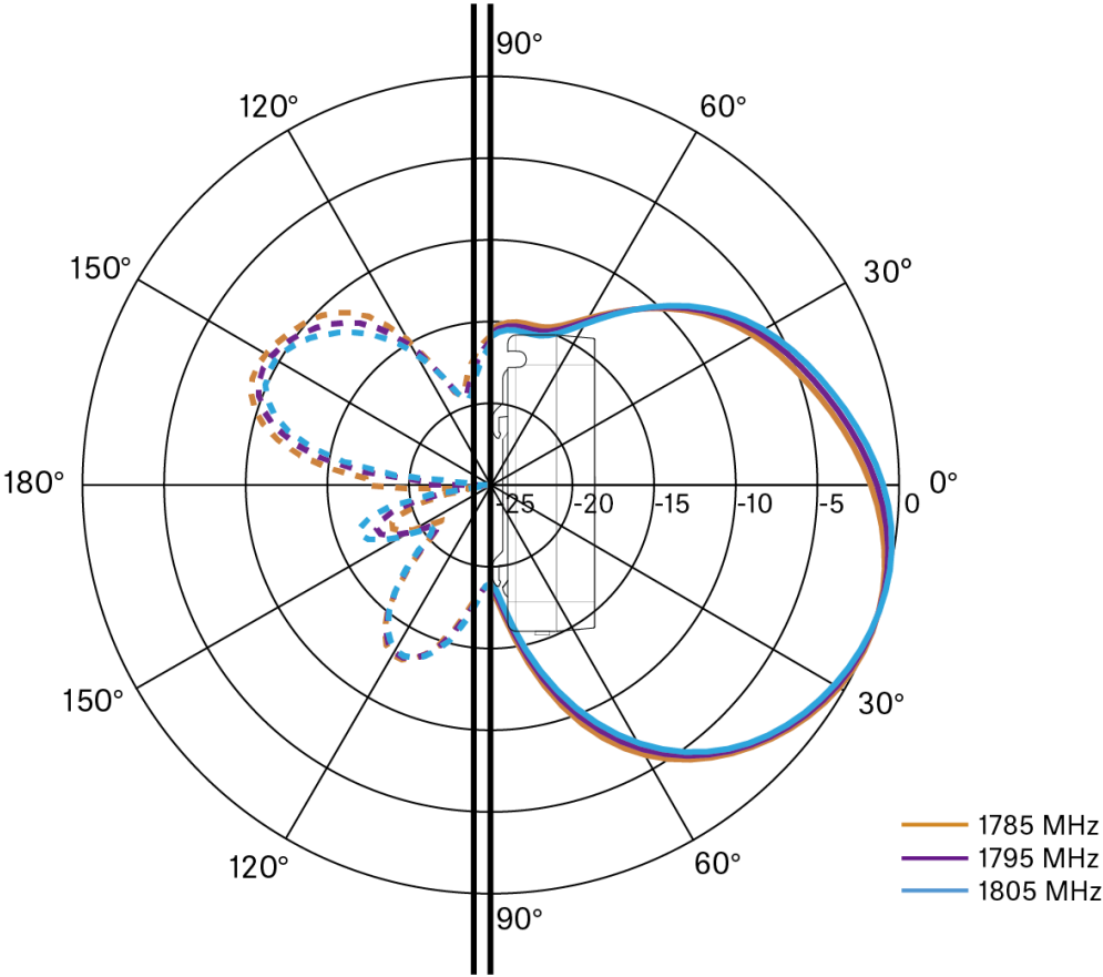
1G8 Vertikal [dB]
