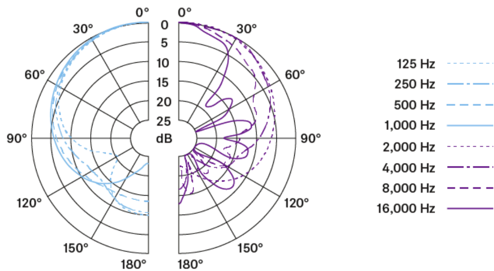
Polardiagramm
