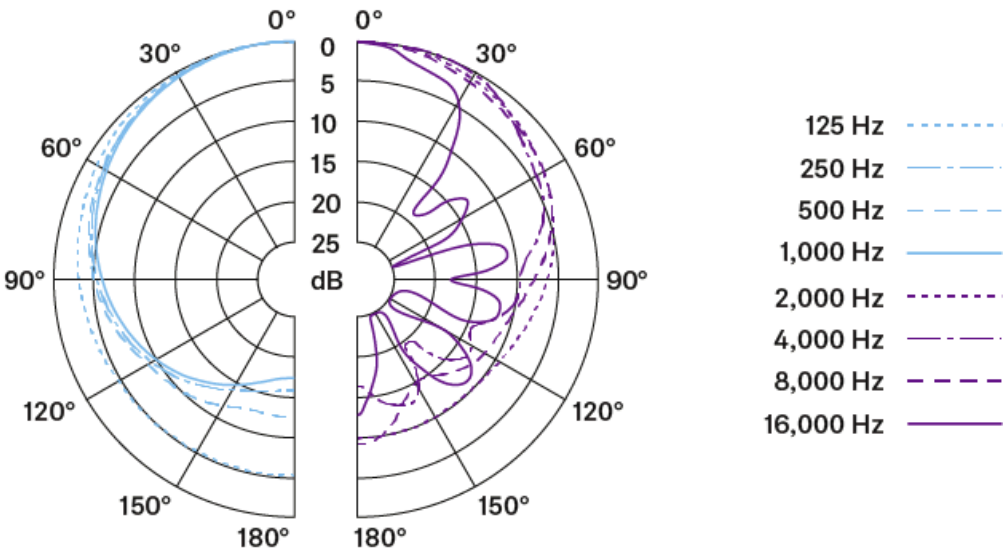
Polardiagramm
