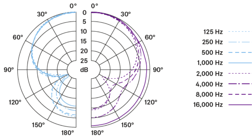
Polardiagramm
